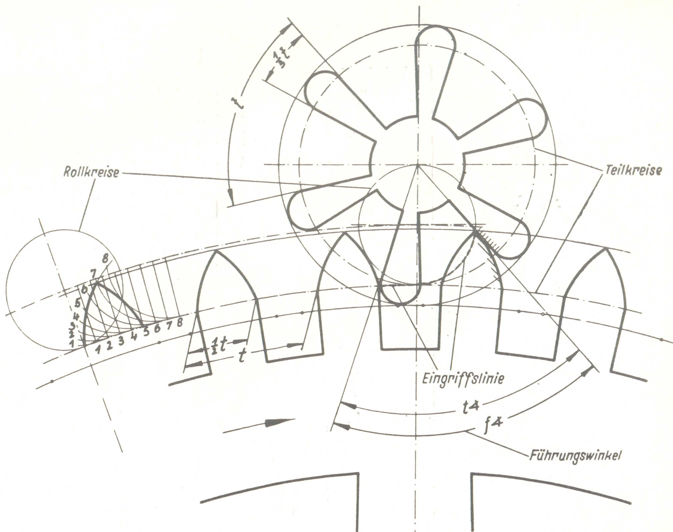
Abb. 52. Entwicklung der Rad- und Triebzahnformen.
